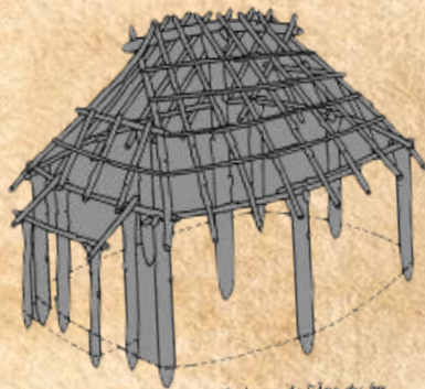
Cabane de l'Age du fer. Reconstitution, plan et coupes.
